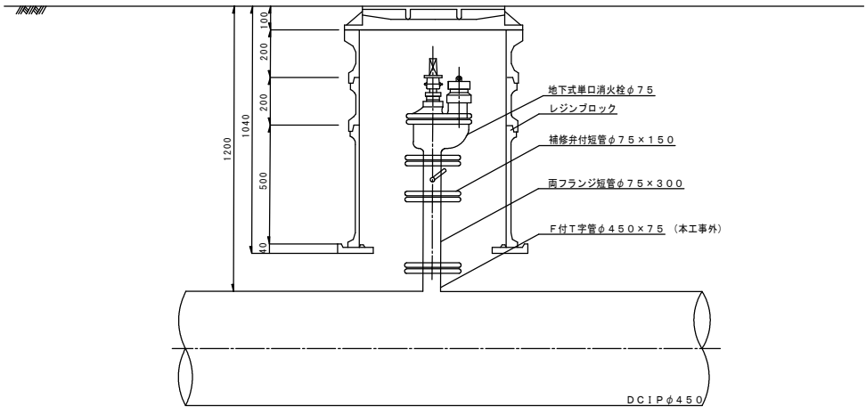
断面図
