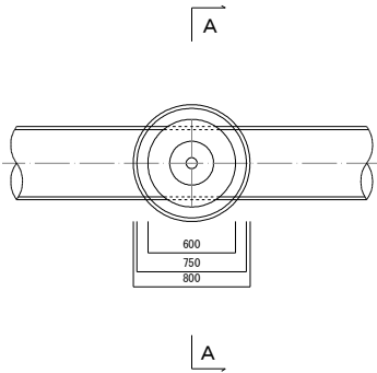
平面図
