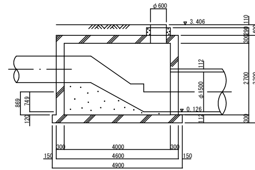
A-A断面図
