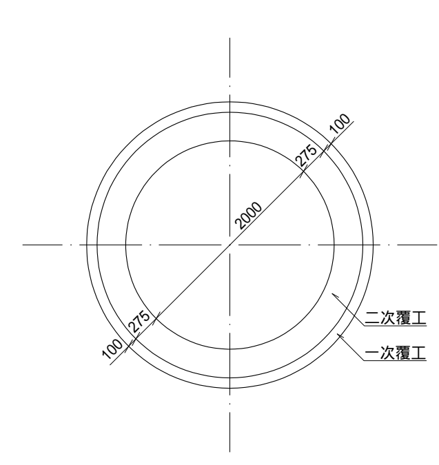
管渠断面図
