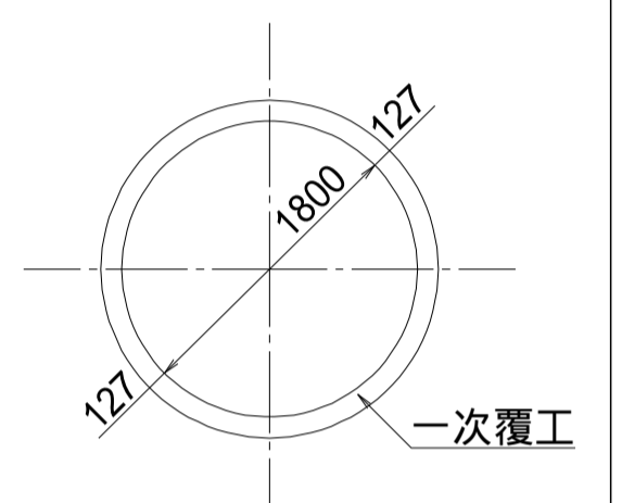
管渠断面図
