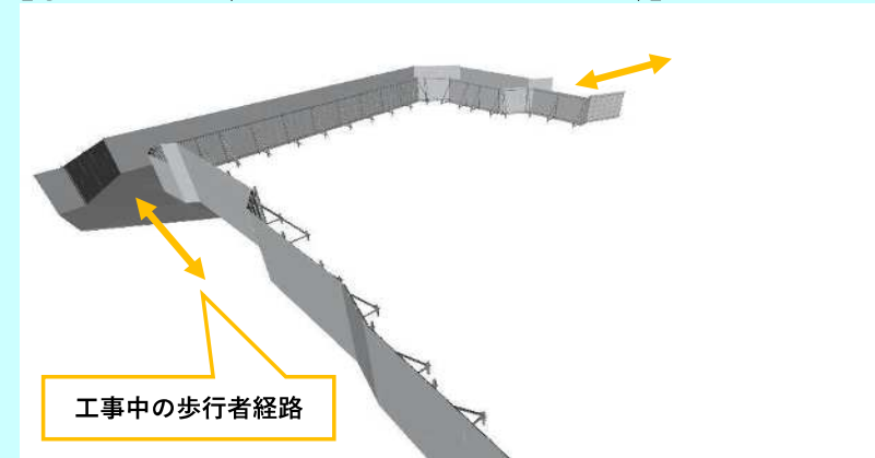
【②工事施工中(歩道切換：仮設歩道切り回し)】
