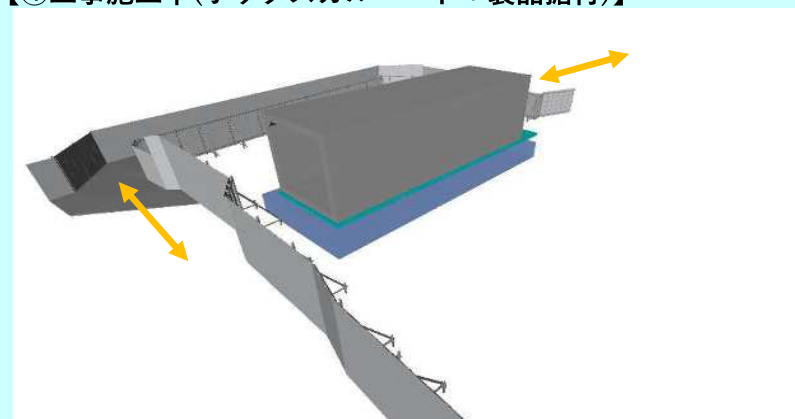
【④工事施工中(ボックスカルバート：製品据付)】
