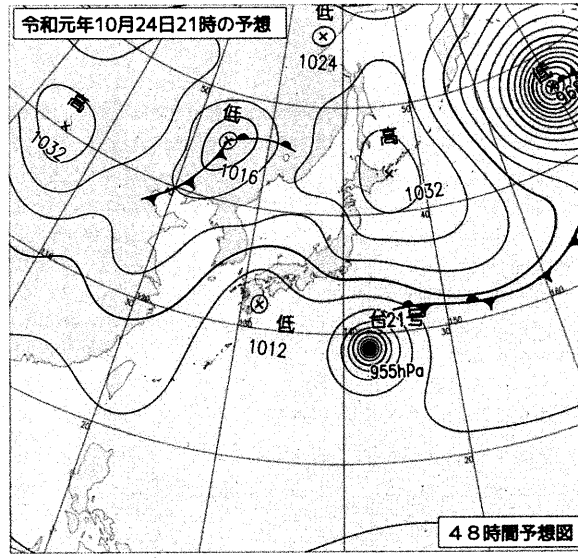
予想地上天気図(10月24日21時)
