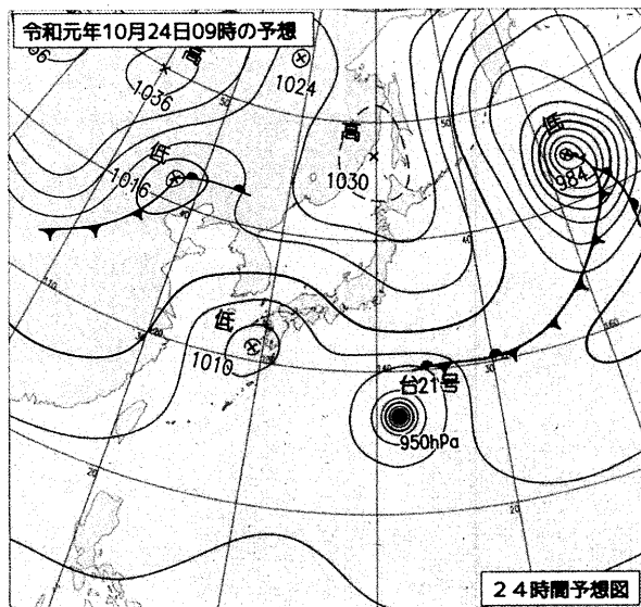
予想地上天気図(10月24日9時)
