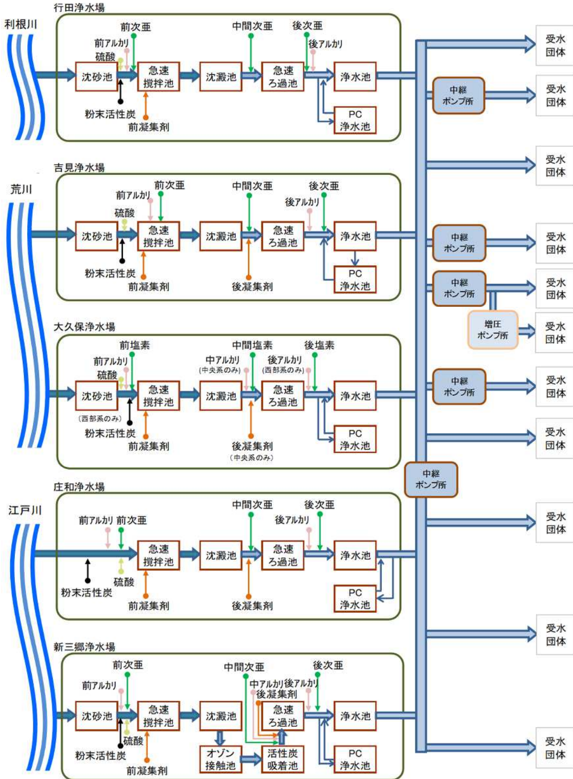
図3 県営水道のフローチャート
