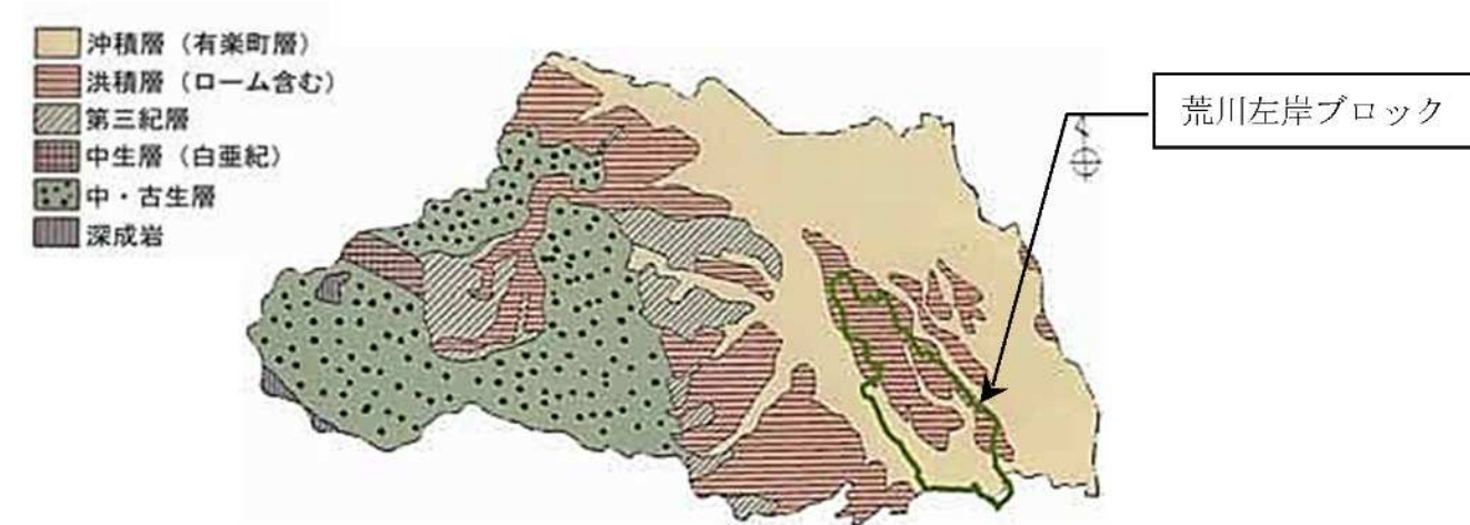
図 1.1.3 埼玉県地質図
