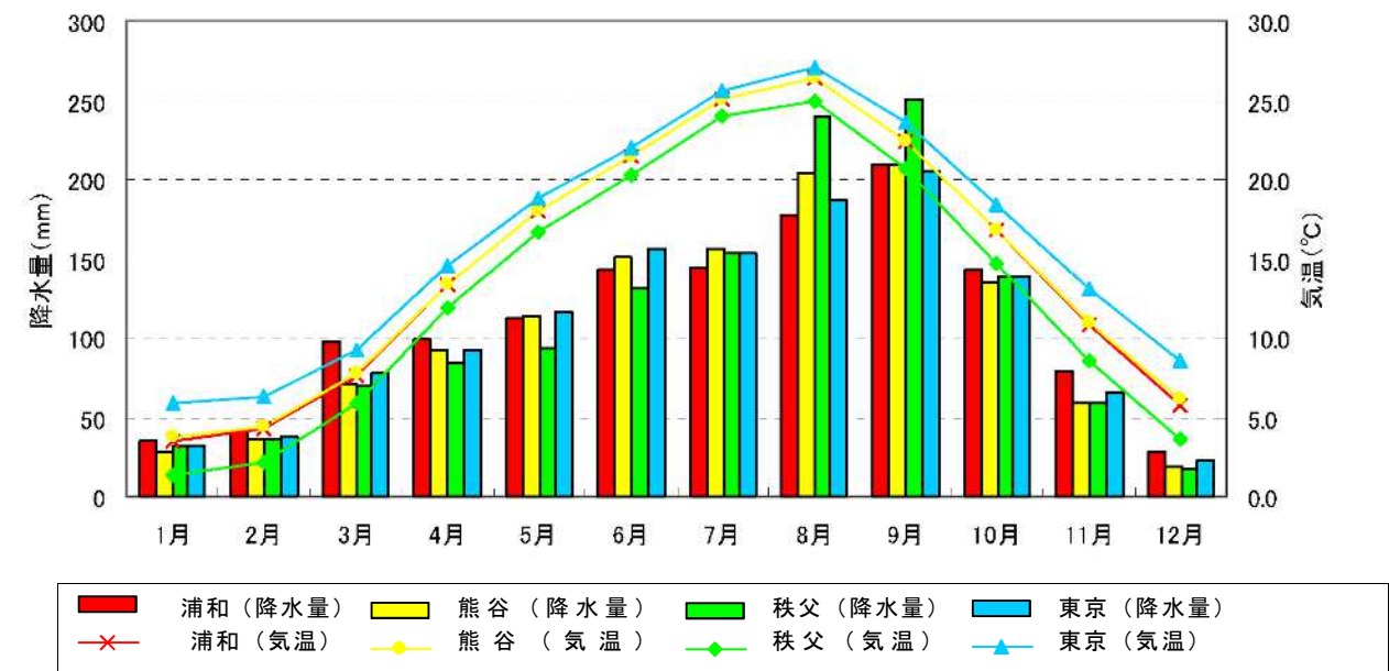
図 1.1.4 月別降水量と月別平均気温 (出典：気象庁アメダス年報)
