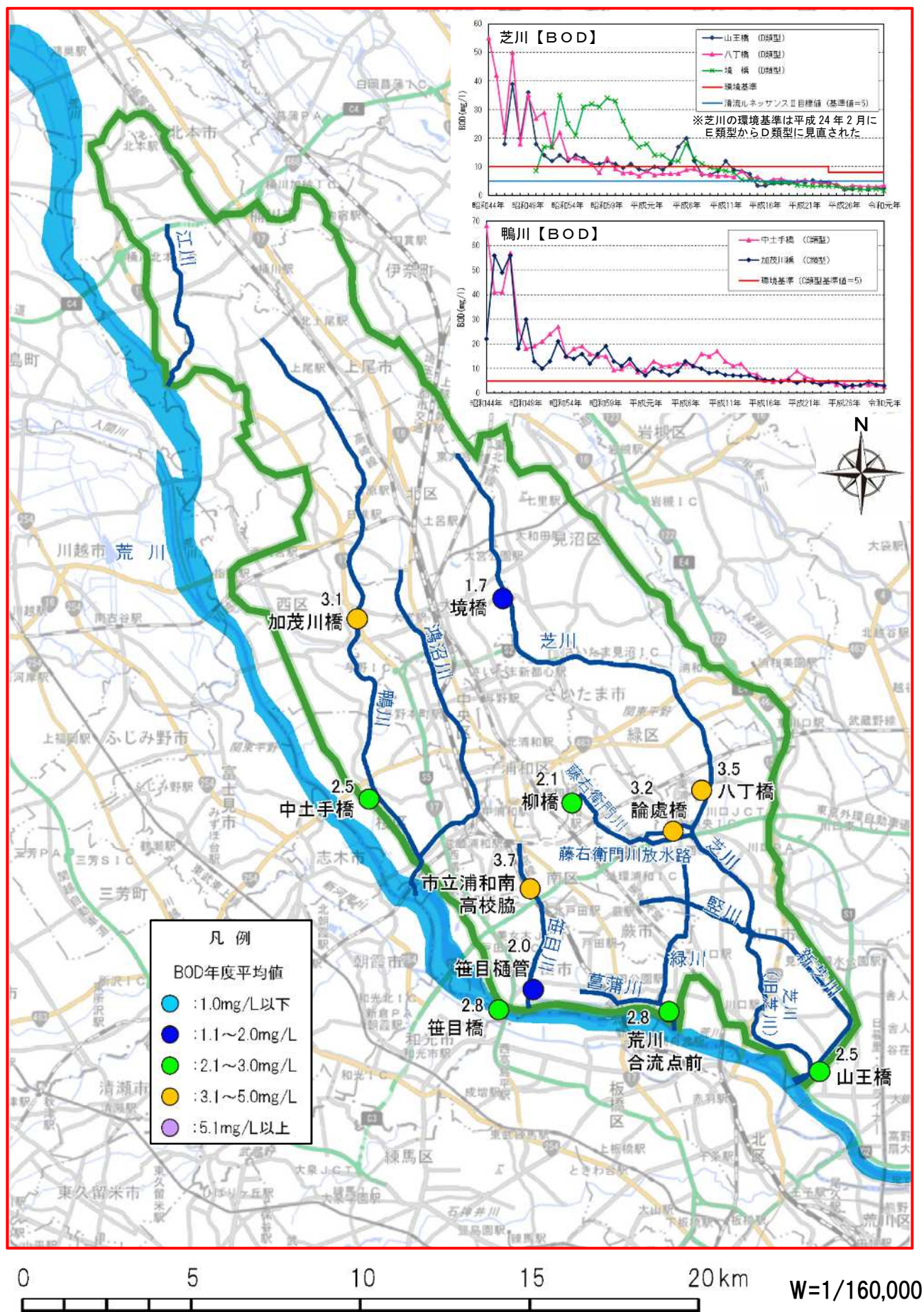
図 1.2.5 荒川左岸ブロック内の水質測定値(令和元年度・BOD 平均値)
