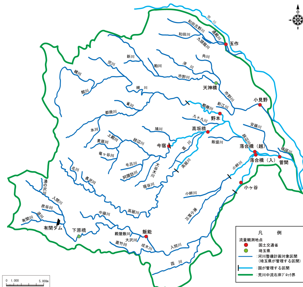
図 1.11 荒川中流右岸ブロックにおける流量観測地点
