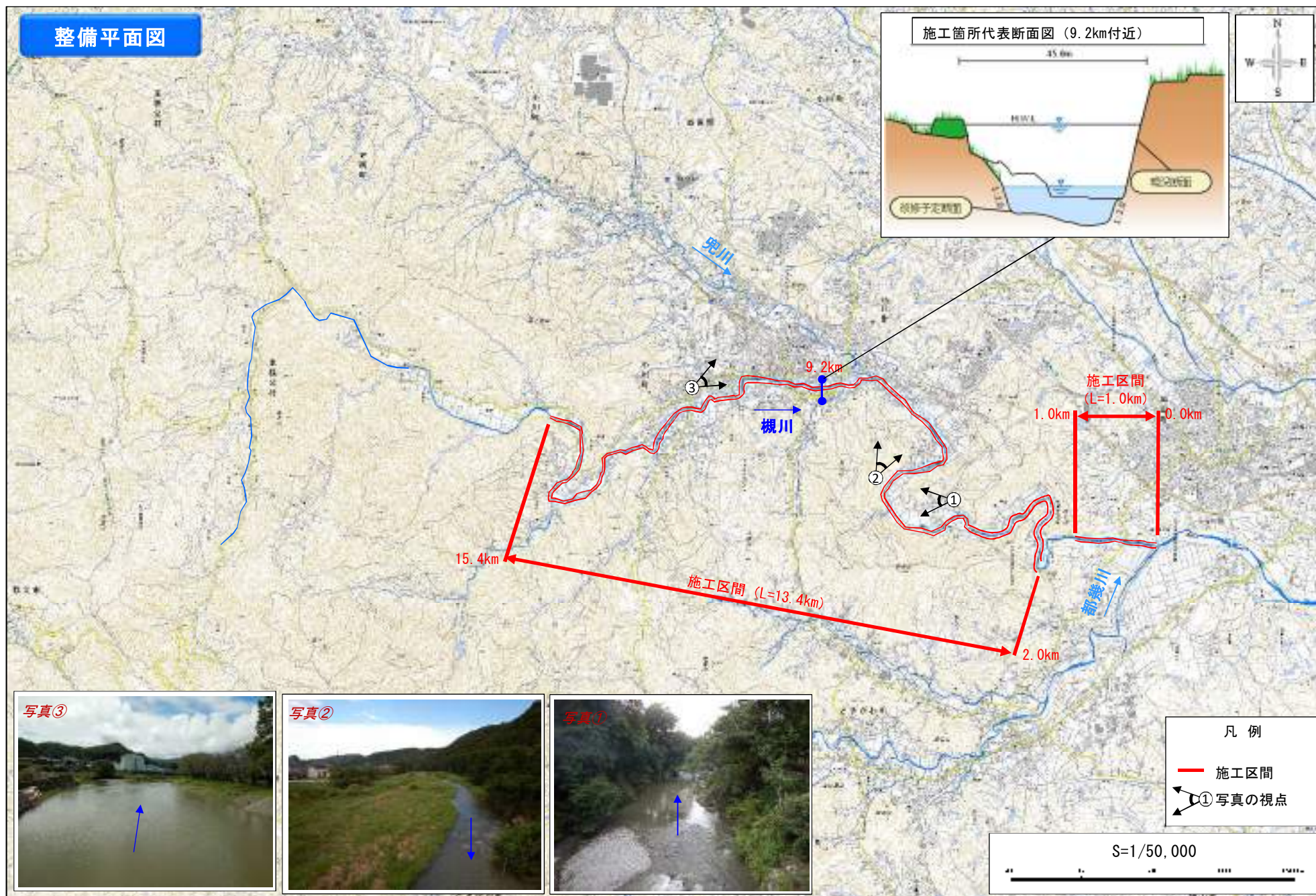
槻川整備平面図 S=1/50,000
