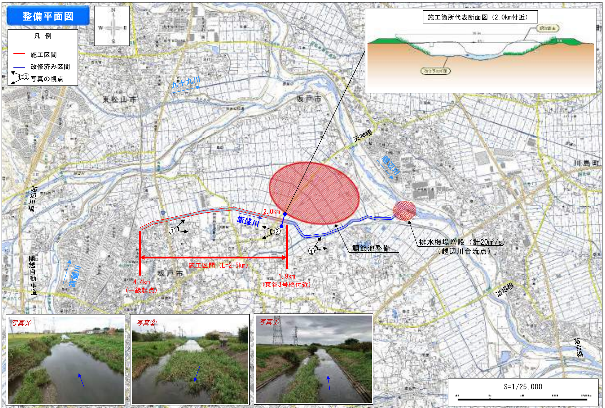
飯盛川整備平面図 S=1/25,000
