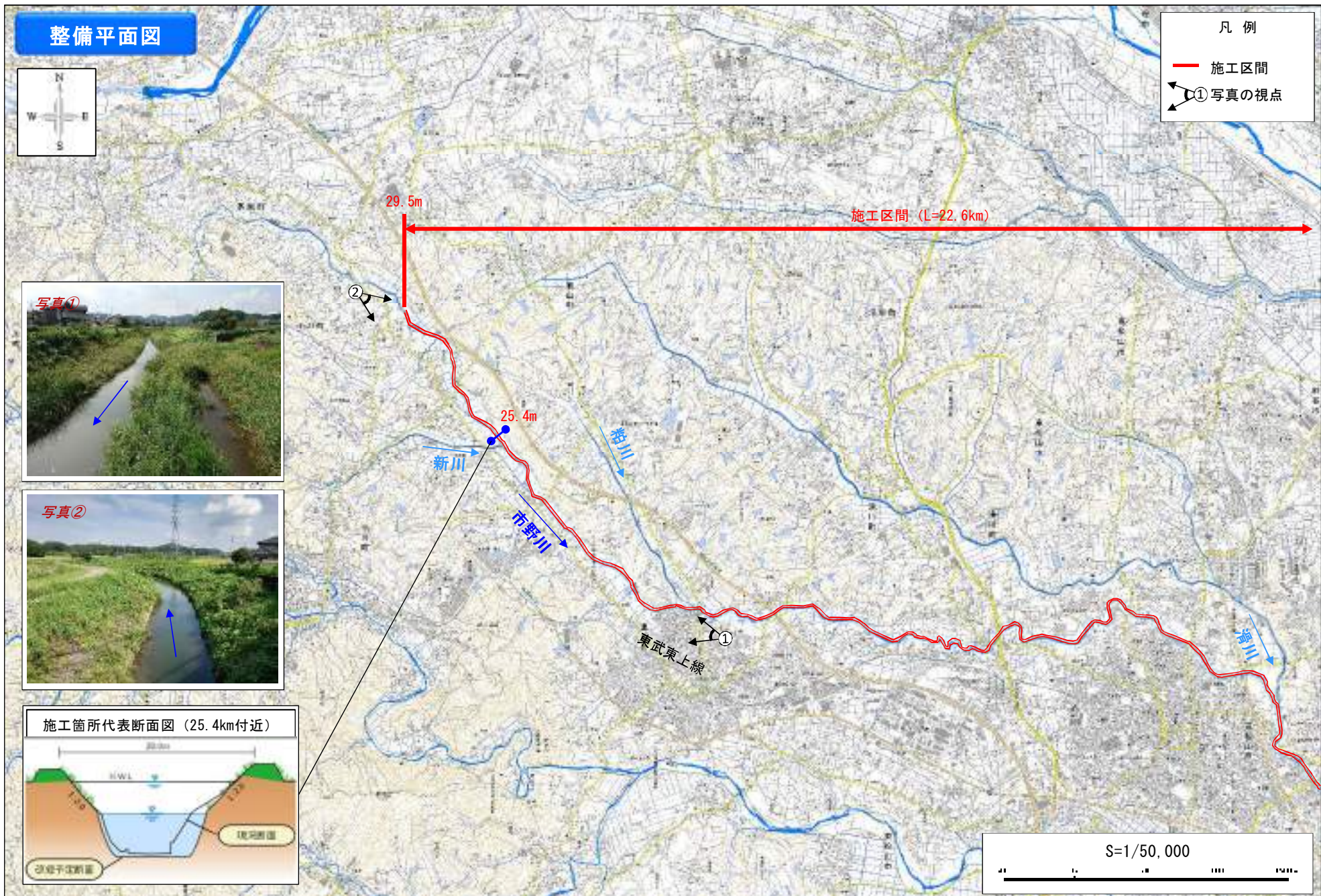
市野川整備平面図1/3 S=1/50,000
