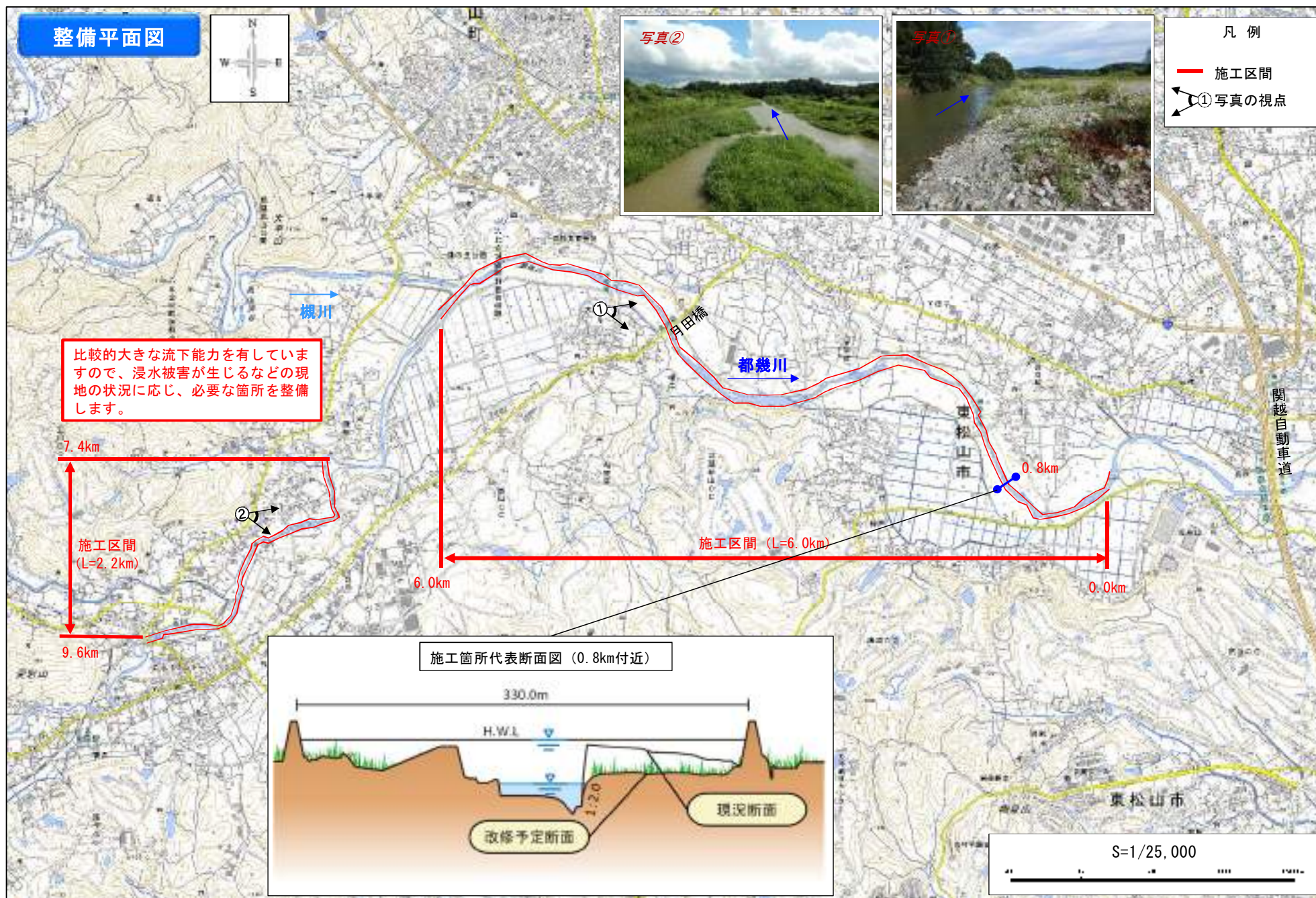
都幾川整備平面図 S=1/25,000
