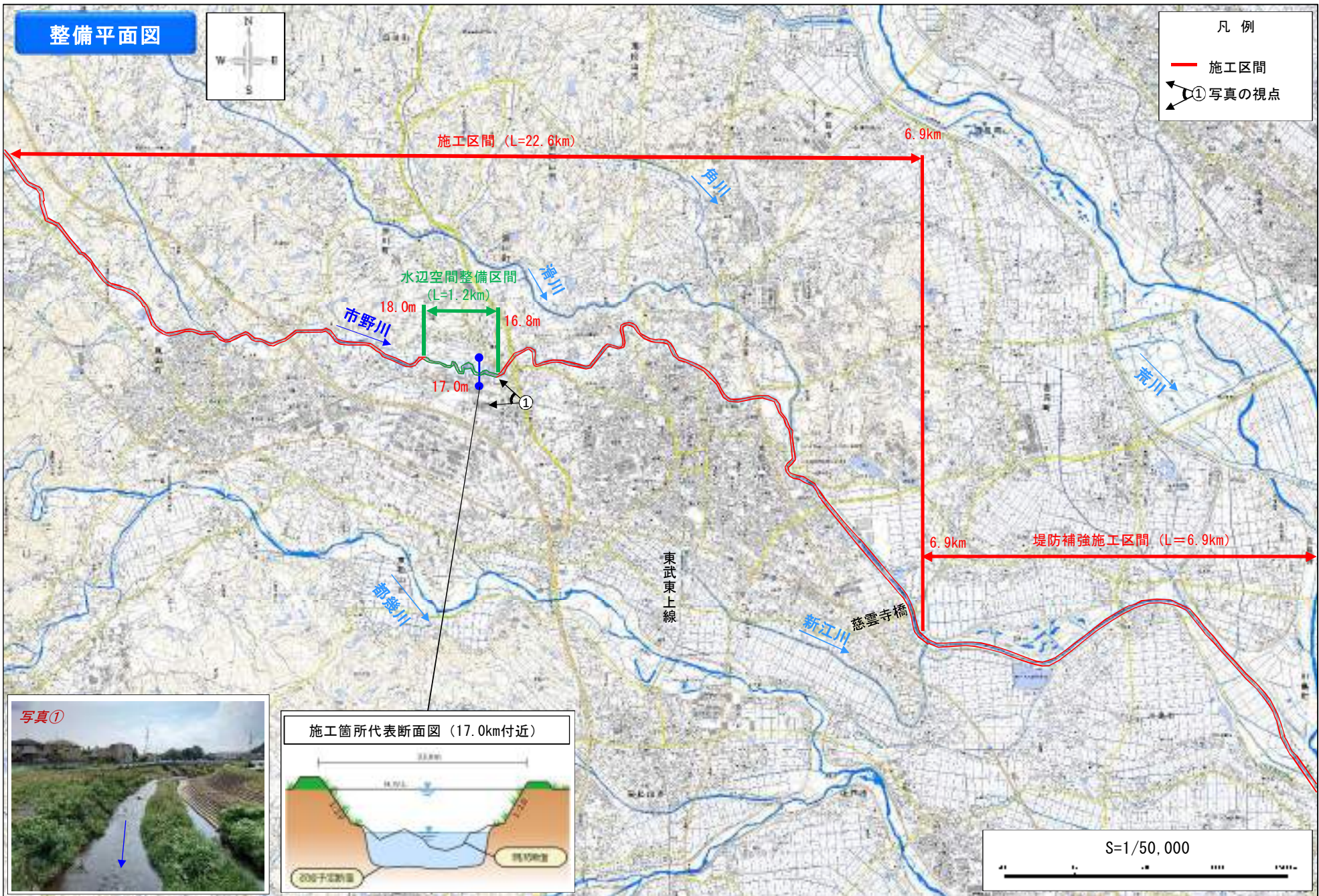
市野川整備平面図2/3 S=1/50,000
