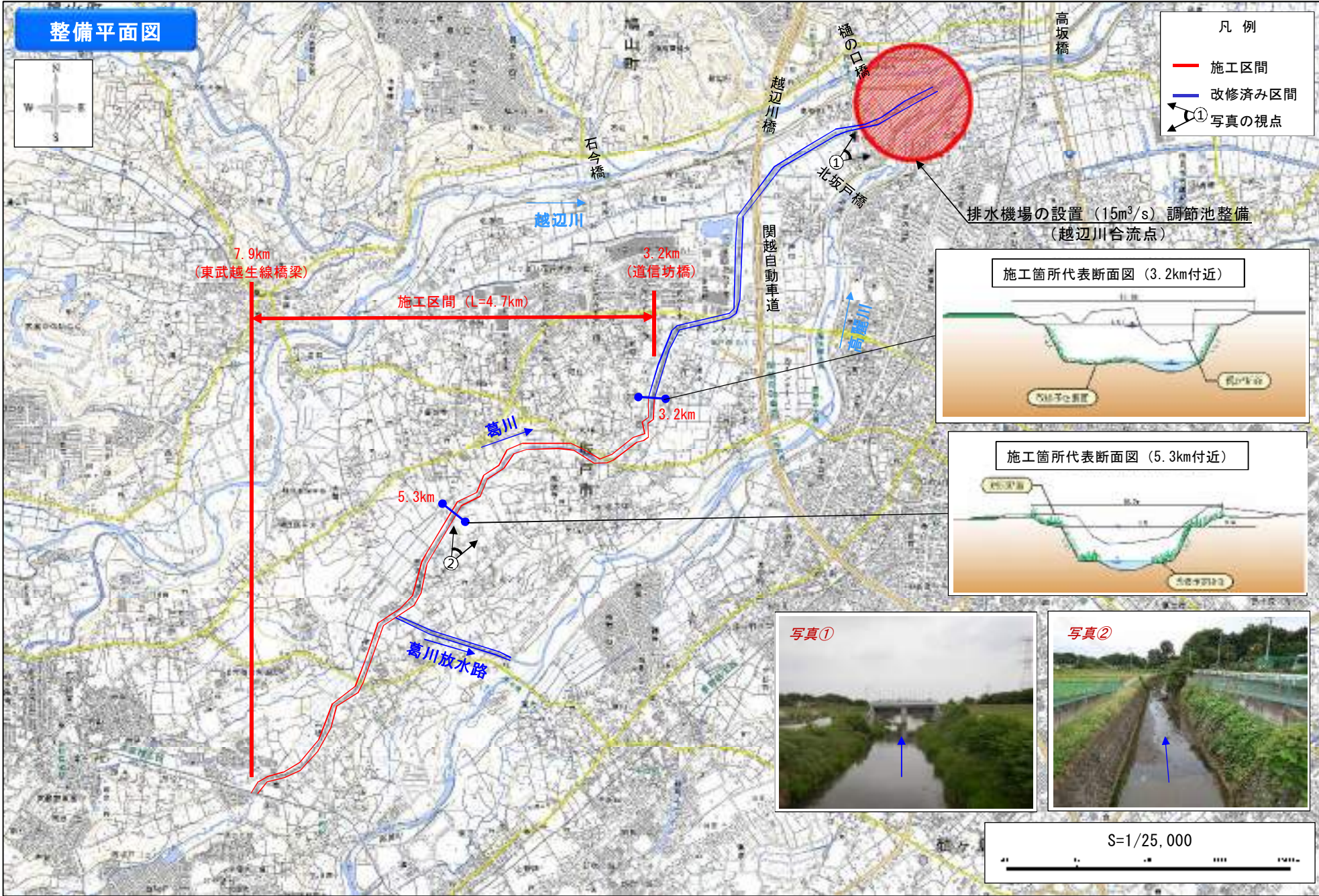
葛川整備平面図 S=1/25,000
