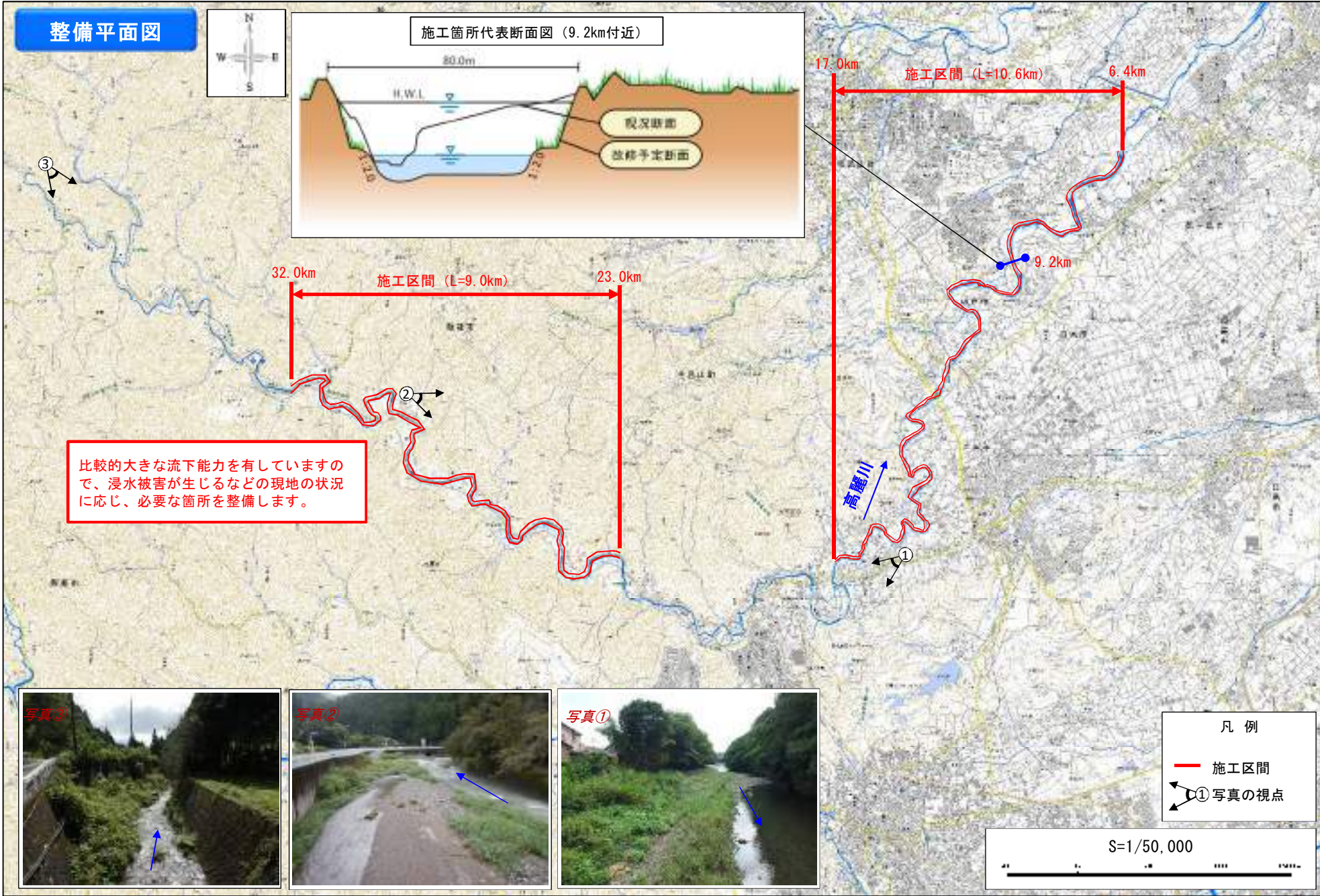
高麗川整備平面図 S=1/50,000
