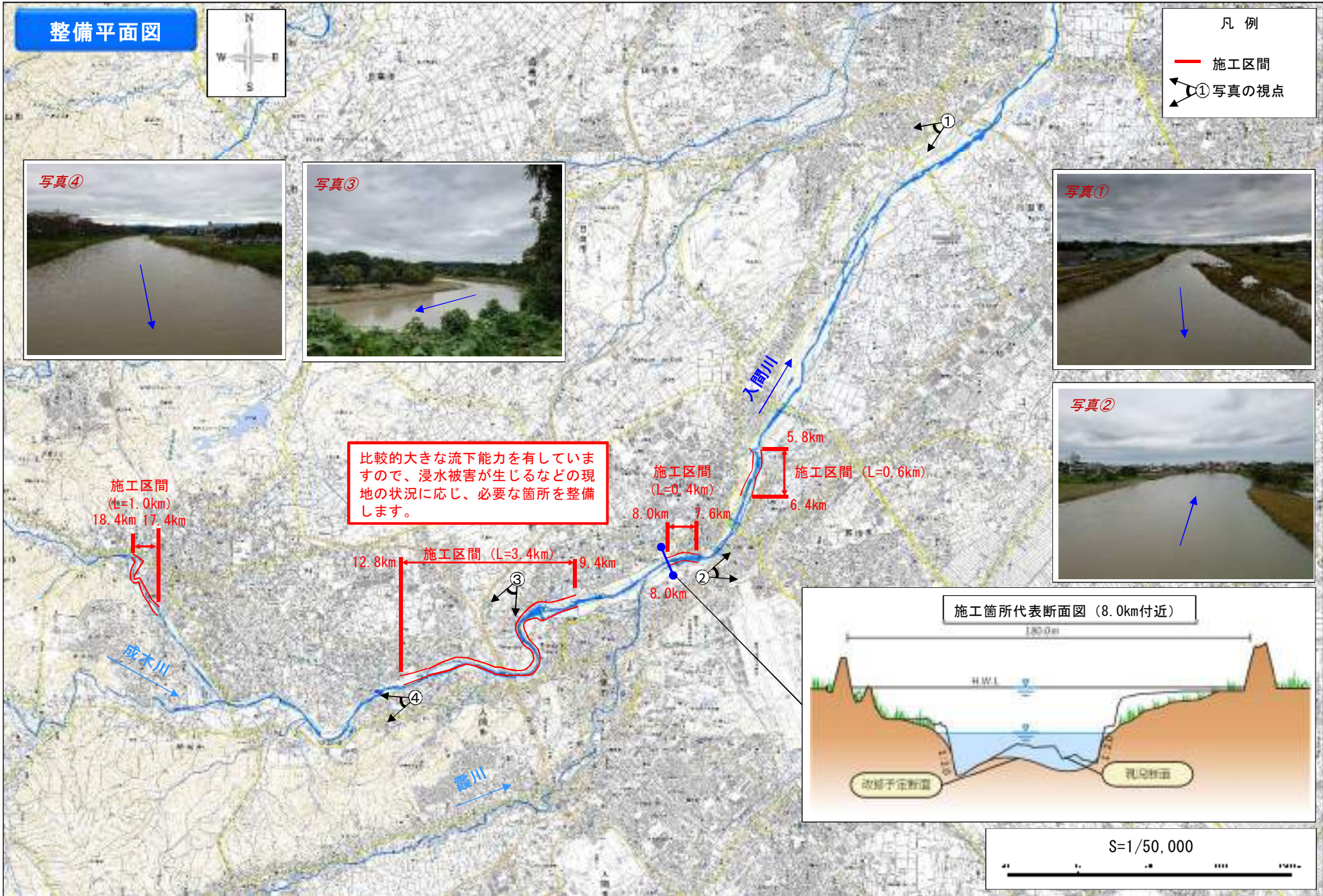
入間川整備平面図2/2 S=1/50,000
