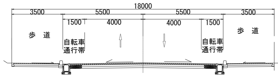
計画道路の横断面図
