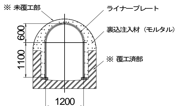
標準断面図
