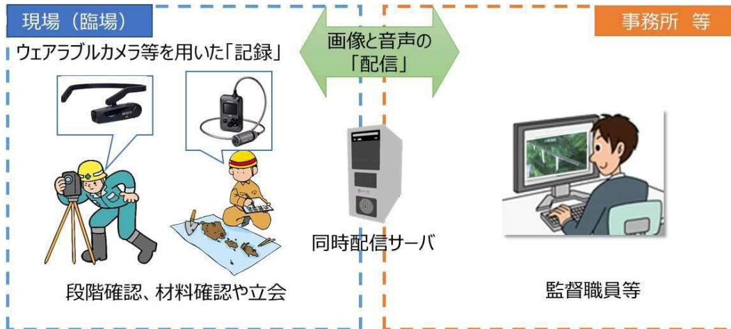
図 2-1 機器構成（例）
