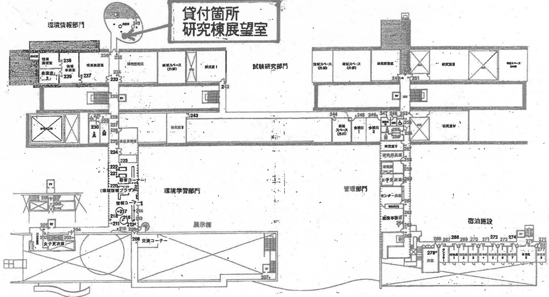
建物平面図
