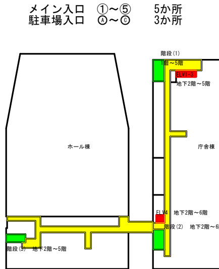
4階平面図
