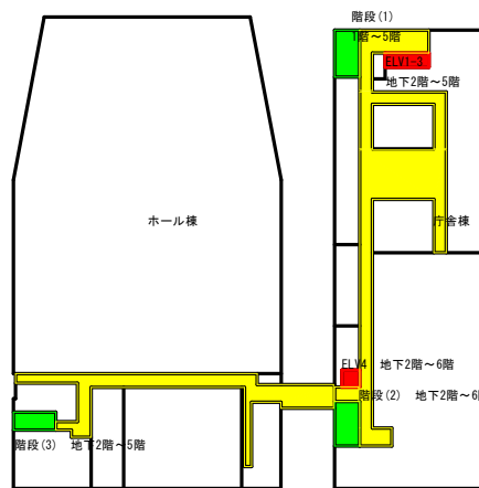
3階平面図
