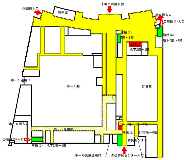
1階平面図
