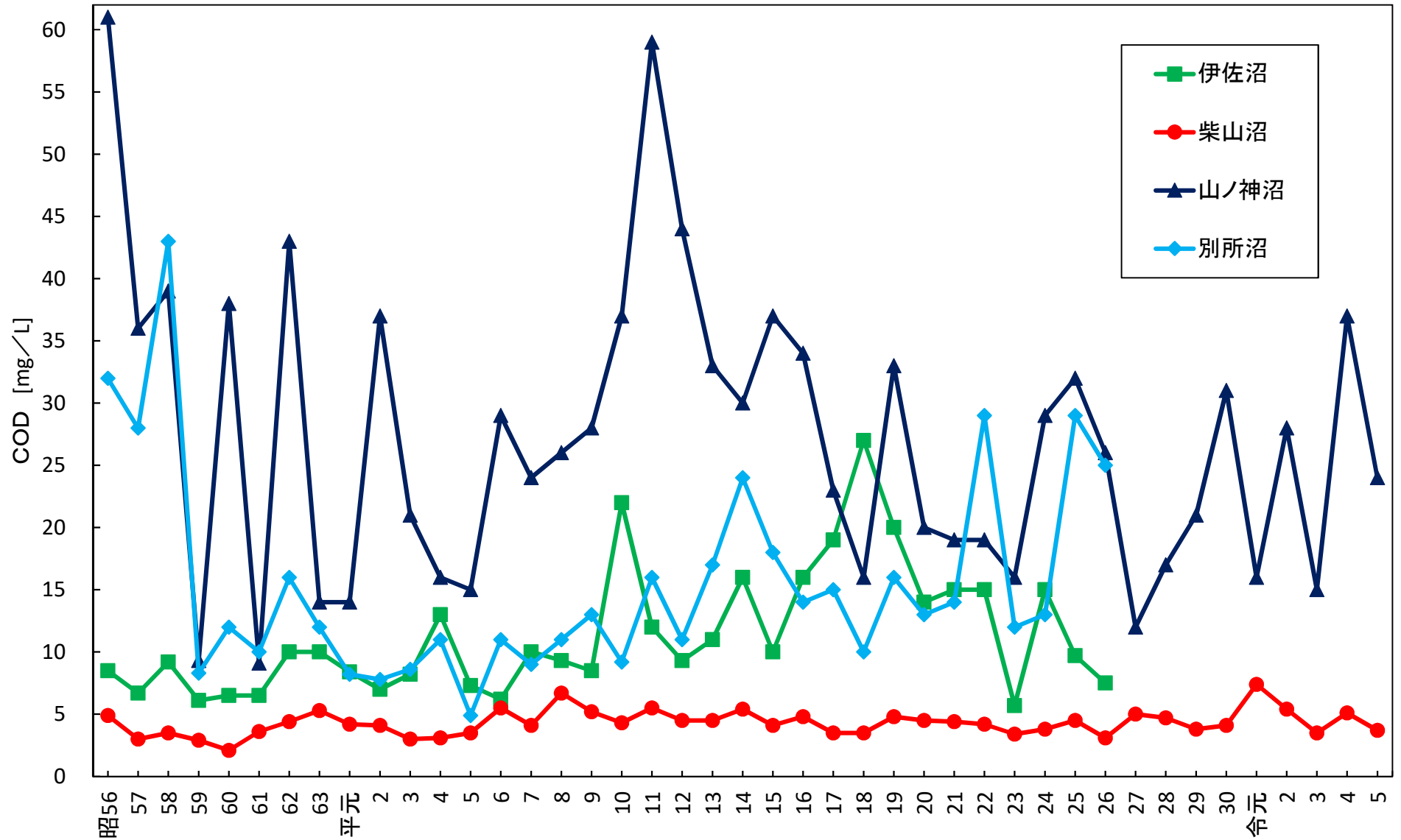
湖沼表層水のCOD経年変化（天然湖沼・夏季）
