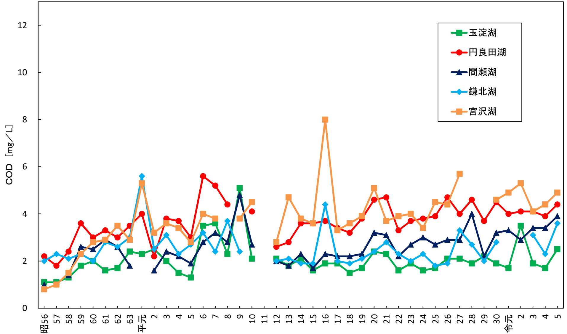
湖沼表層水のCOD経年変化（人工湖沼・冬季）
