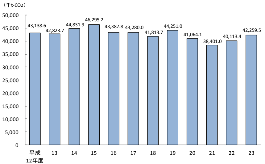
温室効果ガス排出量の推移(県全体)
