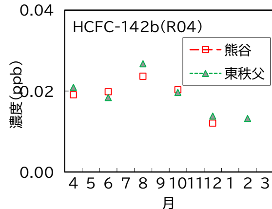
図17 HCFC-142b 濃度の経月変化
