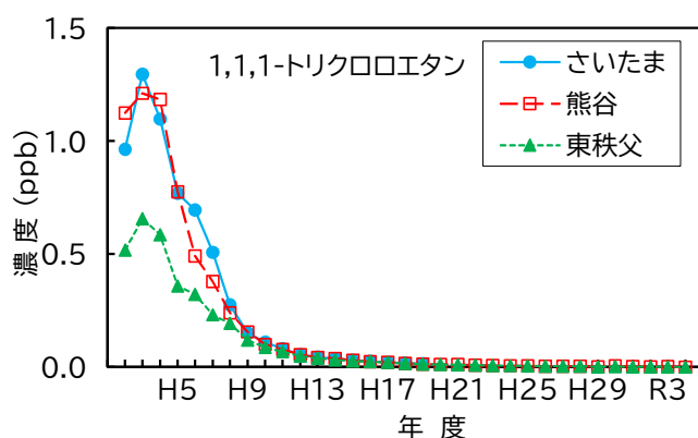
図8 1,1,1-トリクロロエタン濃度の経年変化
