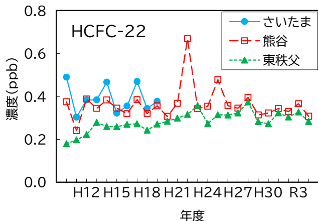
図12 HCFC-22 濃度の経年変化
