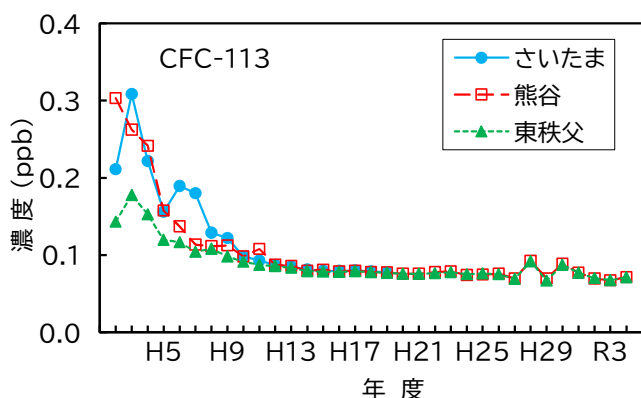
図6 CFC-113濃度の経年変化
