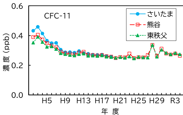
図2 CFC-11濃度の経年変化
