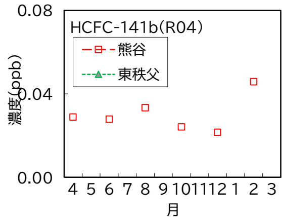
図15 HCFC-141b 濃度の経月変化
