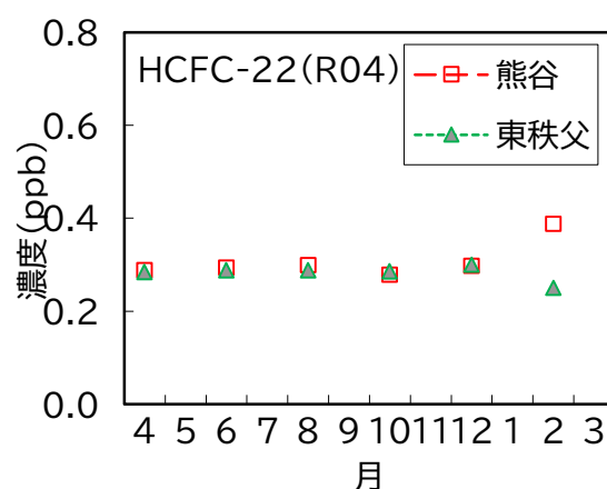
図13 HCFC-22 濃度の経月変化
