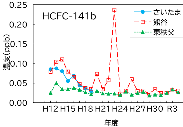
図14 HCFC-141b 濃度の経年変化
