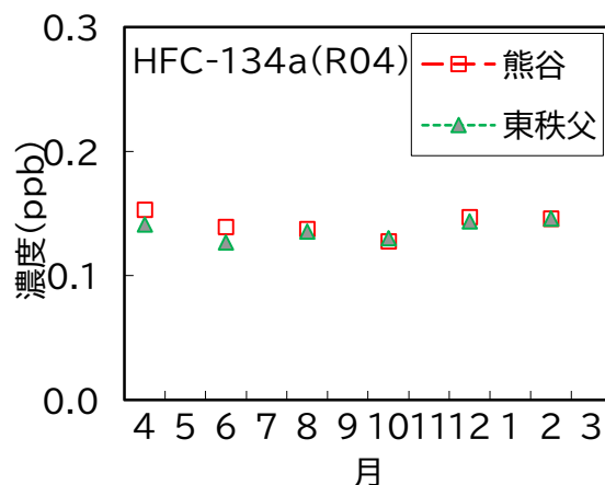
図19 HFC-134a 濃度の経月変化
