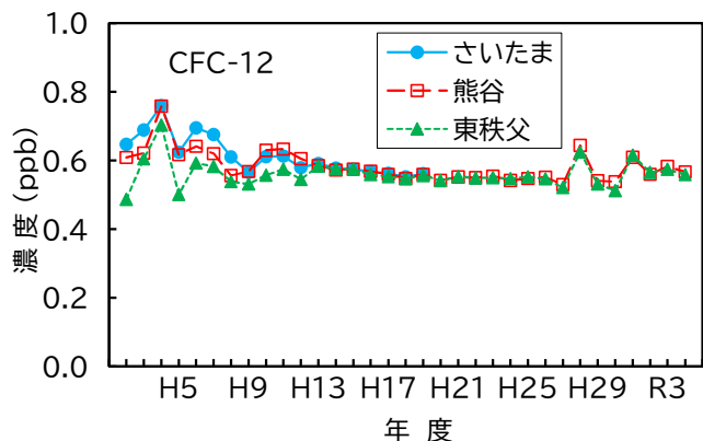
図4 CFC-12濃度の経年変化
