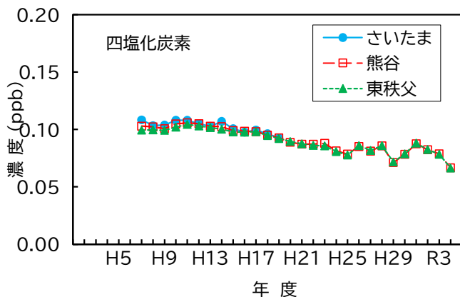
図10 四塩化炭素濃度の経年変化
