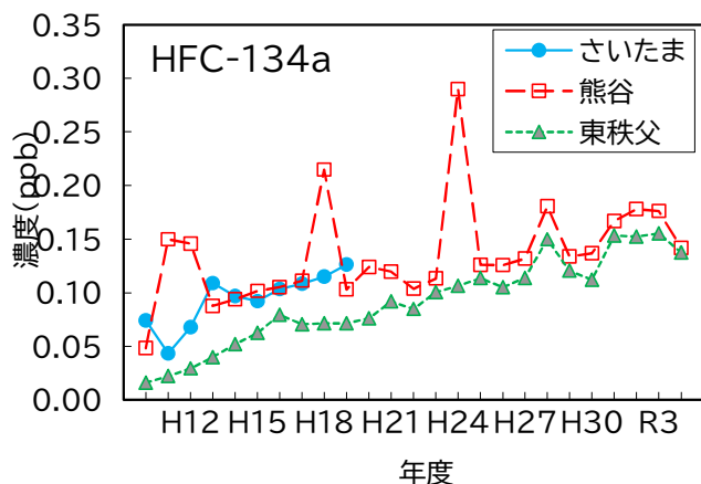
図18 HFC-134a 濃度の経年変化
