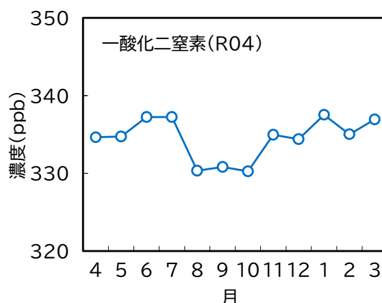
図21 一酸化二窒素濃度の経月変化
