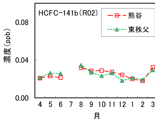
図 15 HCFC-141b 濃度の経月変化
