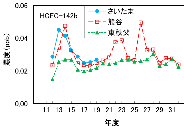
図 16 HCFC-142b 濃度の経年変化
