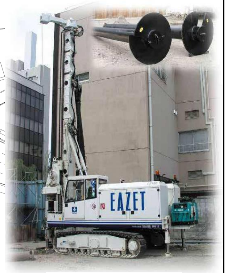
基礎杭施工写真
