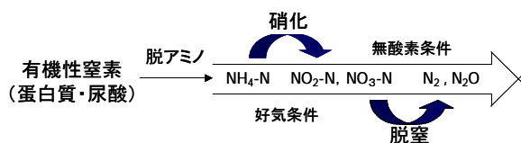
図19 生物学的窒素除去の概念
