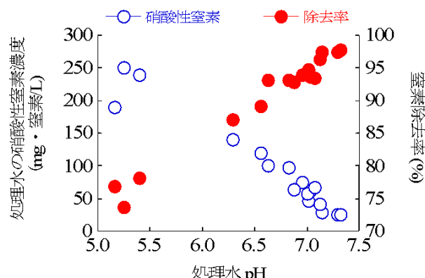
図20 処理水pHと窒素除去率の関係
