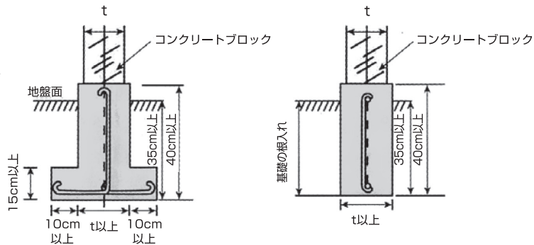
軟弱地盤の場合
