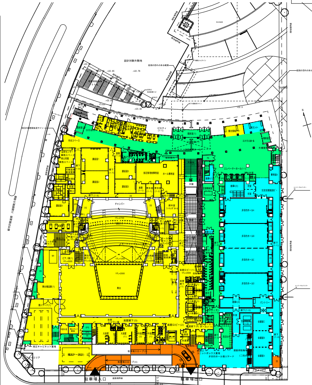
市道1526号線 1階平面図 Scale:1/600
